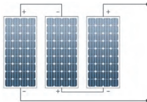
شکل ۱۶- اتصال سری
