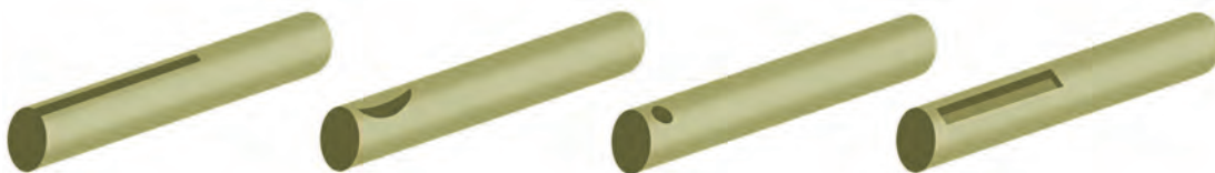
شکل ۸۰-انواع جای خار روی محورها
