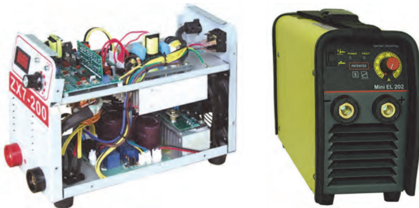
شکل ۱۳- اینورتر جوشکاری و اجزای داخلی آن
