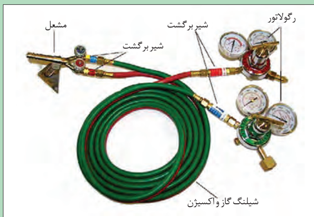
شکل ۱۸- محل نصب سوپاپ های یک طرفه (شیر برگشت)
