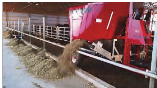
فیدر میکسر در حال تخلیه مواد
