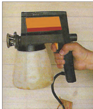
شکل ۶۱- پیستوله بدون کمک هوای فشرده (Airless)
