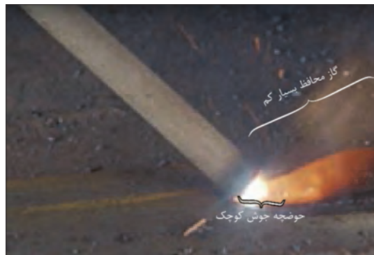
شکل ۲۶- جوشکاری با آمپر بسیار پایین
